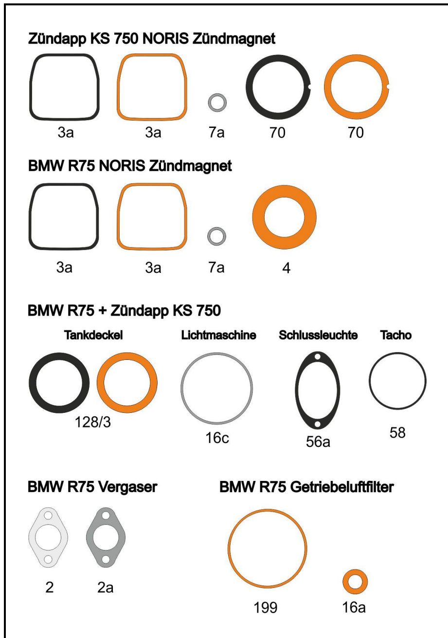
Tafel 53: Dichtungen BMW R75 + Zündapp KS 750
